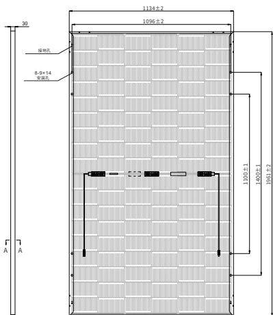
产品图示 单位: mm
